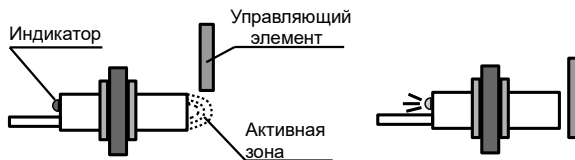
Рисунок 7.1. Работа датчика вращения
