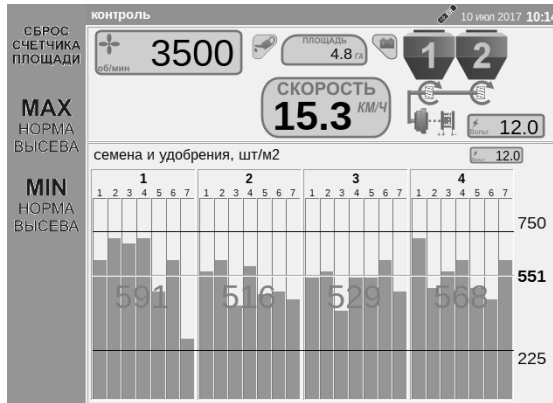
Рисунок 4.1. Диаграмма распределения семян по семяпроводам
